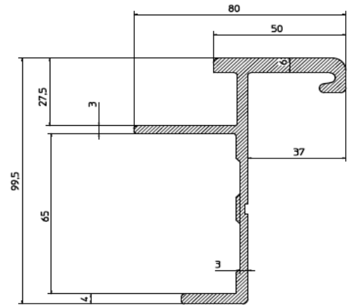
TS11 2.427 kg/m
