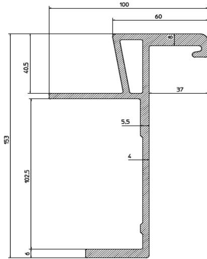
TS10 4.537 kg/m
