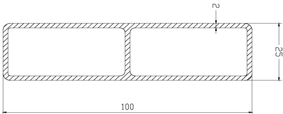
ATP135 1.411 kg/m
