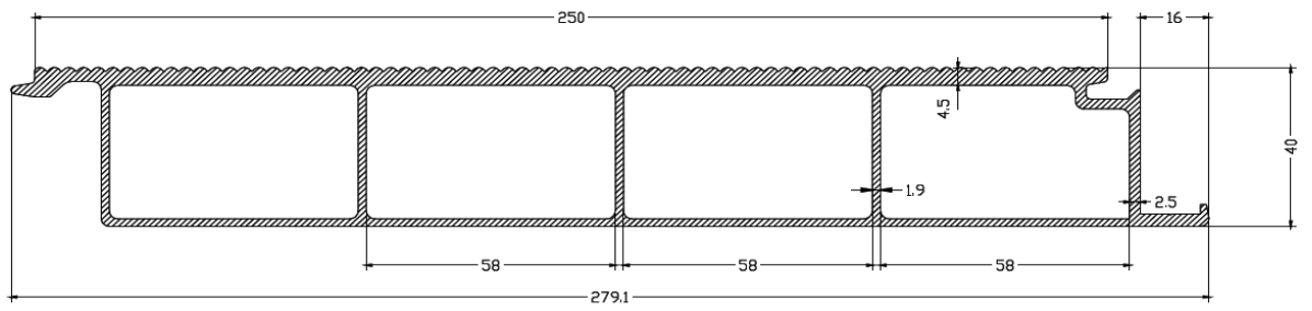
TS11 2.427 kg/m
