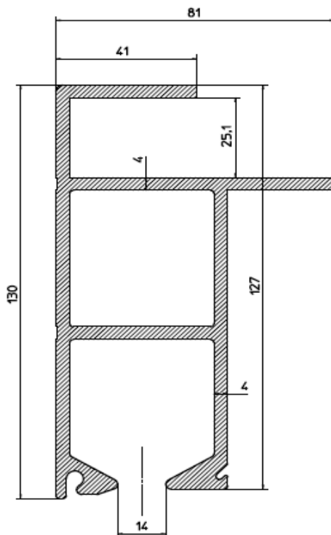
TS12 4.516 kg/m
