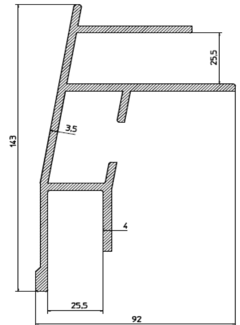
TS13 3.517 kg/m
