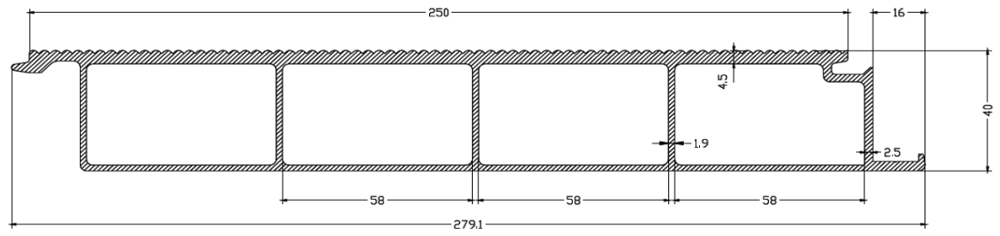
TS11 2.427 kg/m
