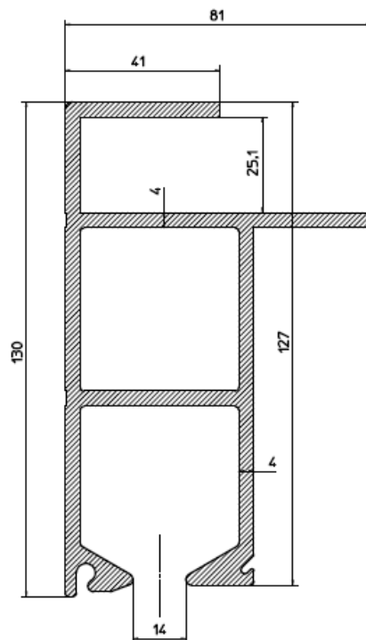
TS12 4.516 kg/m
