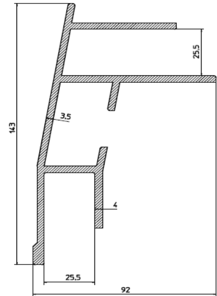
TS13 3.517 kg/m
