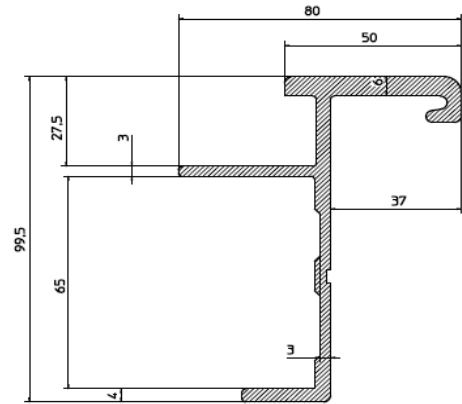
TS11 2.427 kg/m
