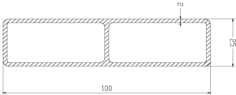
ATP135 1.411 kg/m
