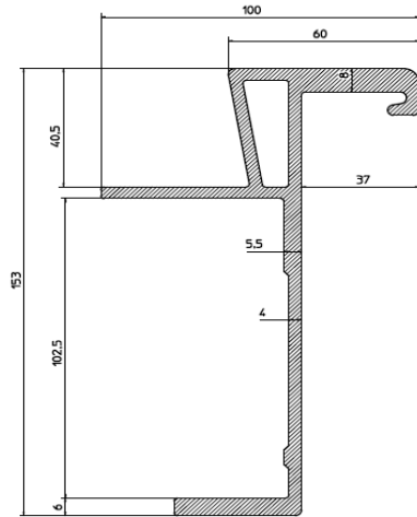
TS10 4.537 kg/m
